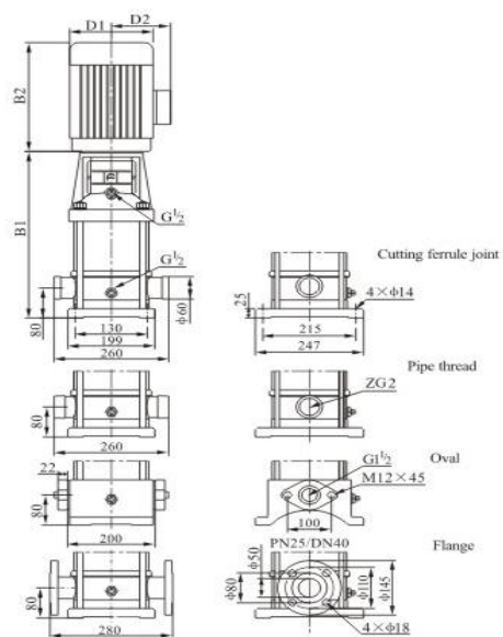
Model Size(mm) Weight (Kg) B1 B2 B1+B2 D1 D2 CDLF8 CDLT8-2/1 347 245 592 170 142 32 CDLF8 CDLT8-2 357 290 647 190 155 38 CDLF8 CDLT8-3 387 290 677 190 155 41 CDLF8 CDLT8-4 427 345 772 197 165 49 CDLF8 CDLT8-5 457 345 802 197 165 50 CDLF8 CDLT8-6 487 355 842 230 188 58 CDLF8 CDLT8-8 567 390 957 260 208 71 CDLF8 CDLT8-10 627 390 1017 260 208 80 CDLF8 CDLT8-12 687 390 1077 260 208 82 CDLF8 CDLT8-14 835 500 1335 330 255 153
