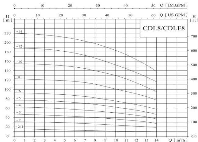
Performance table Model Driving motor Q (m³/h) 7 8 9 10 11 12 13 14 (kw) (hp) CDLF8 CDLT8-2/1 0.75 1 H (m) 13 12 11.5 11 10.5 10 9.5 9 CDLF8 CDLT8-2 1.5 2 27 26 25 24 23 22 20 18 CDLF8 CDLT8-3 2.2 3 41 40 38 37 35 33 30 28 CDLF8 CDLT8-4 3 4 55 54 52 50 47 45 41 38 CDLF8 CDLT8-5 3 4 70 68 65 63 59 56 52 47 CDLF8 CDLT8-6 4 5.5 85 82 78 76 72 68 62 57 CDLF8 CDLT8-8 5.5 7.5 115 110 105 101 97 91 84 75 CDLF8 CDLT8-10 7.5 10 145 140 132 126 122 115 105 95 CDLF8 CDLT8-12 7.5 10 173 167 160 152 147 132 125 115 CDLF8 CDLT8-14 11 15 202 195 188 179 174 163 147 135
